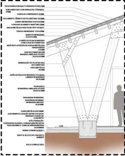
DETALHAMENTO 1 ESC:1/20
